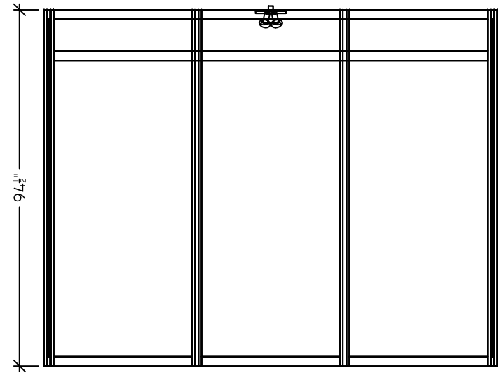
ÉLÉVATION
